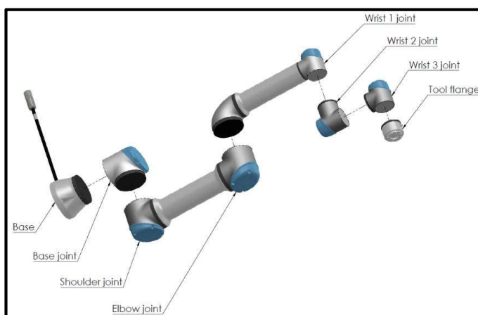
Fig. 9 – Despiece del robot
